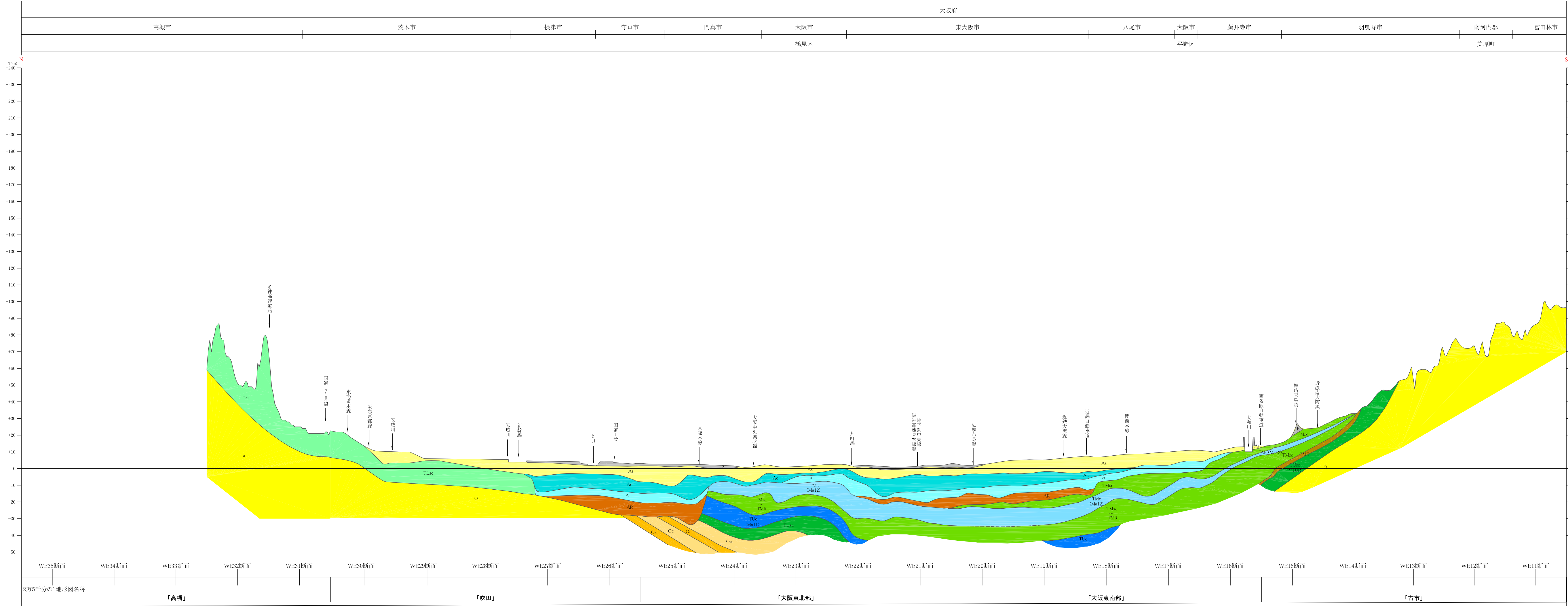
NS14-1断面
