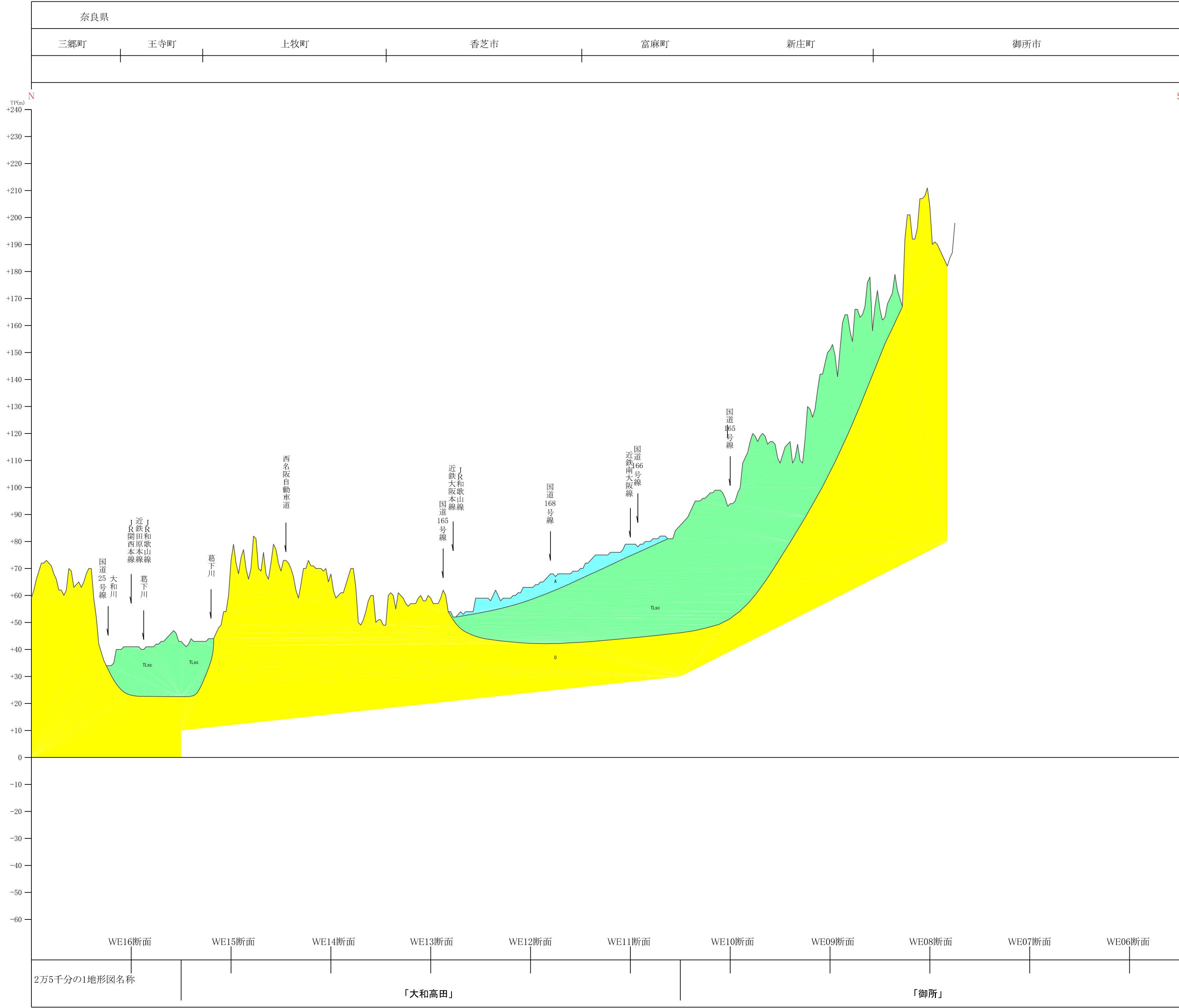
NS19-2断面
