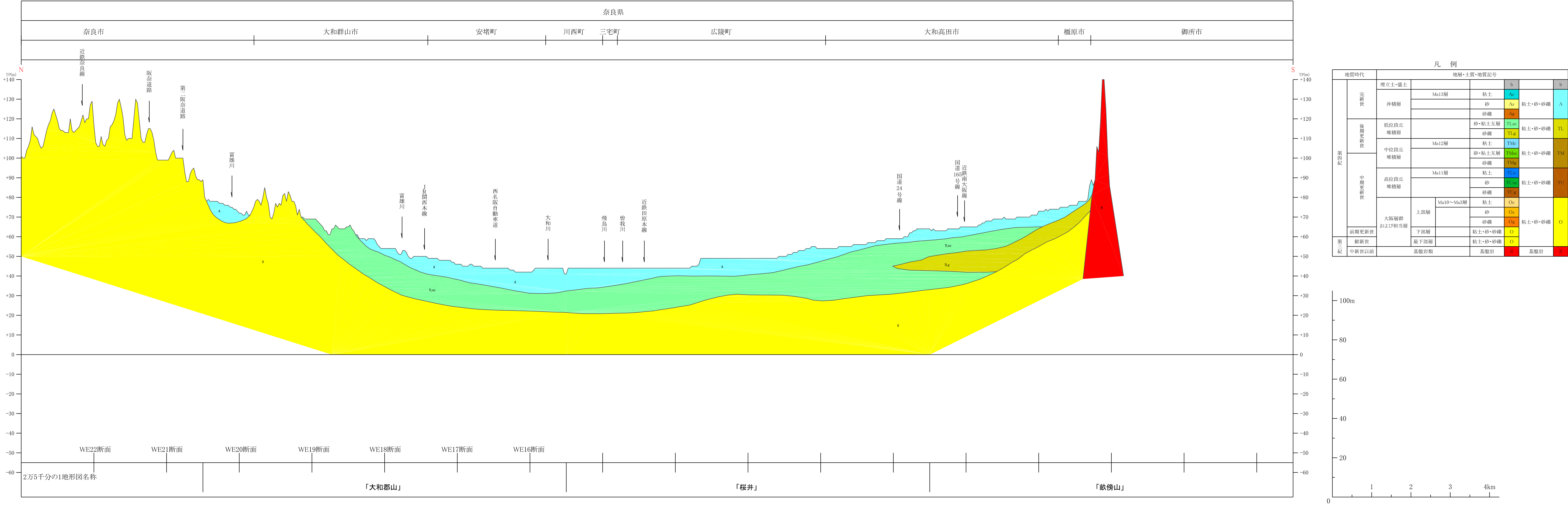
NS21-2断面
