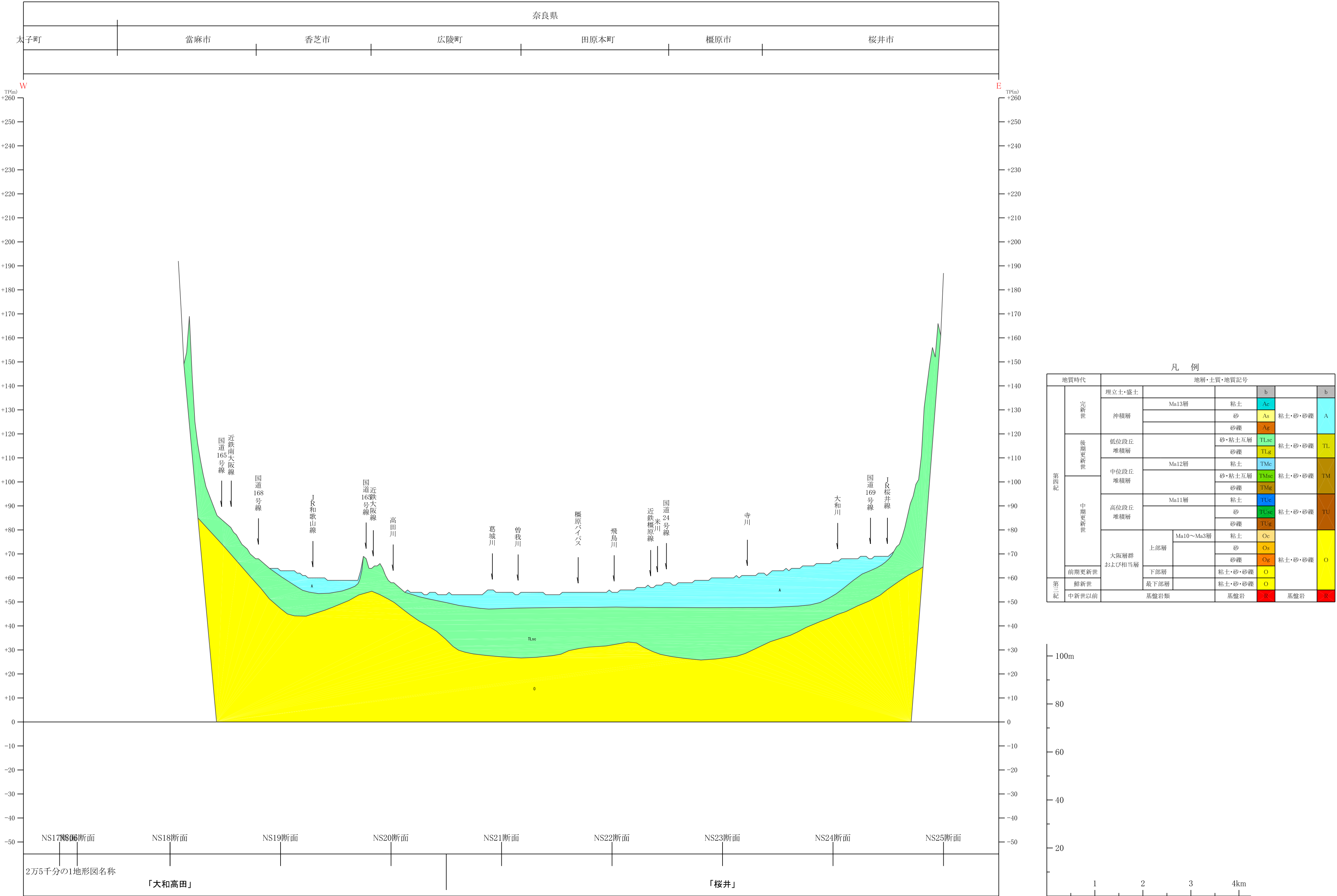
WE12-2断面
