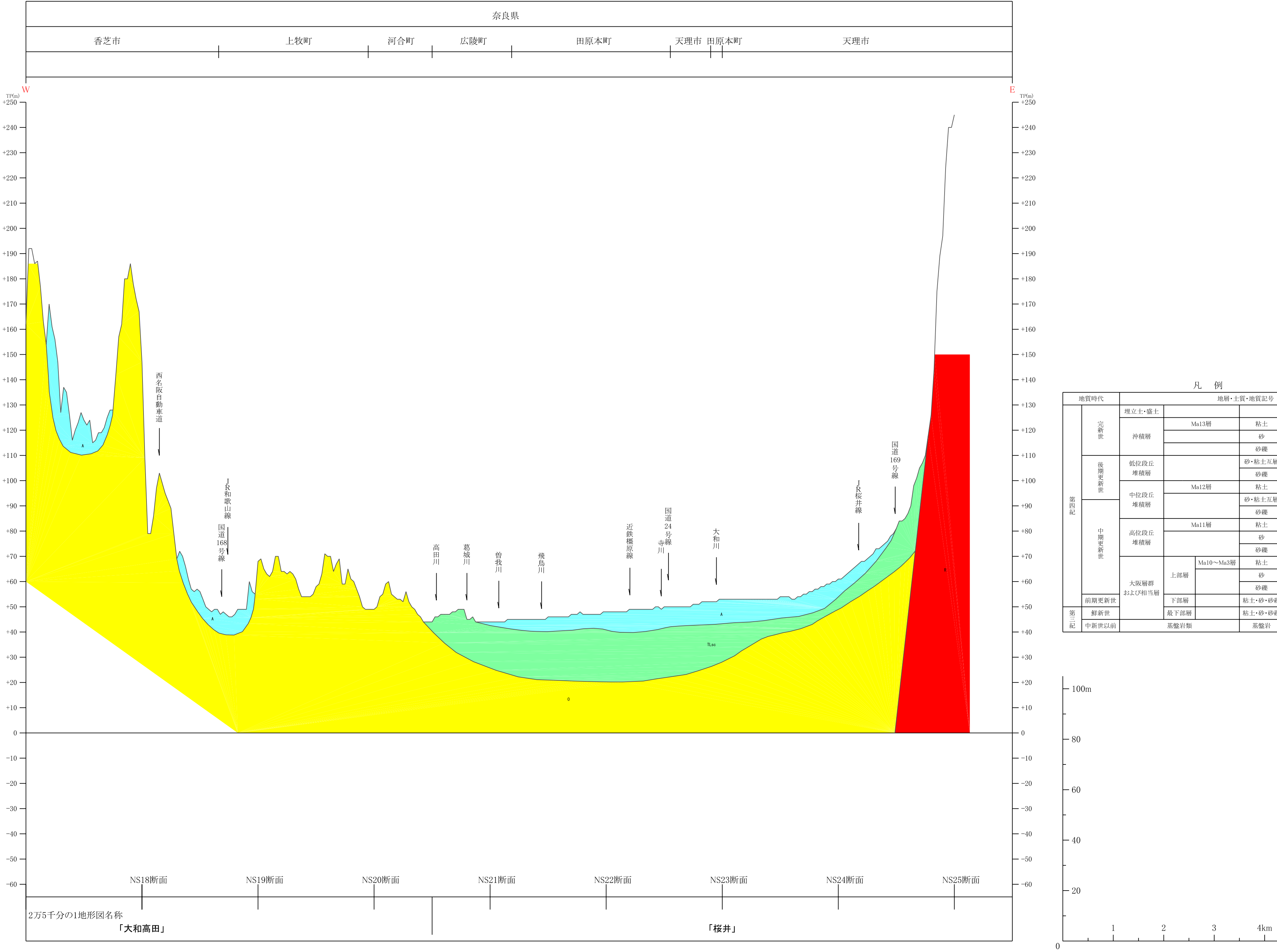
WE14-2断面
