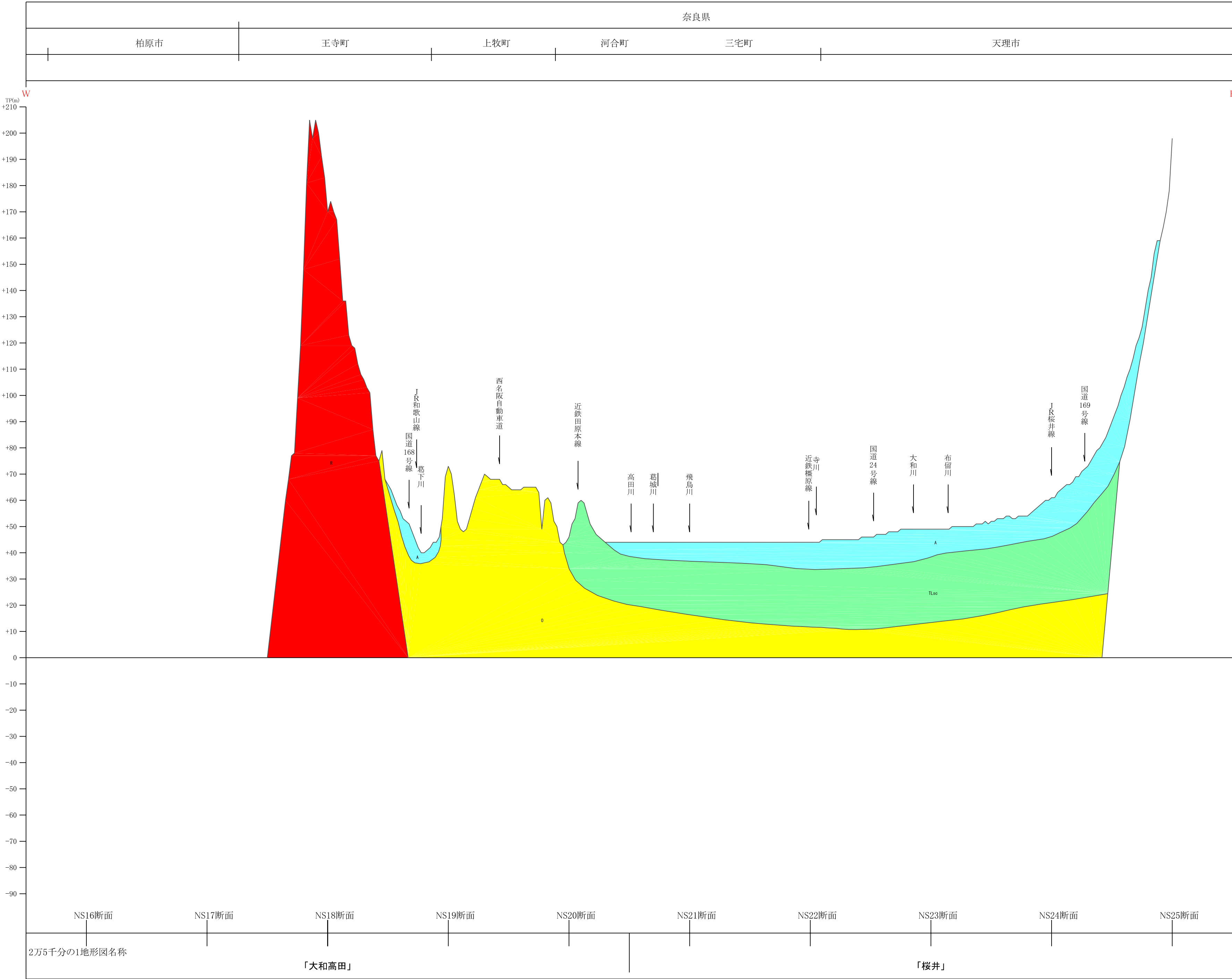
WE15-2断面
