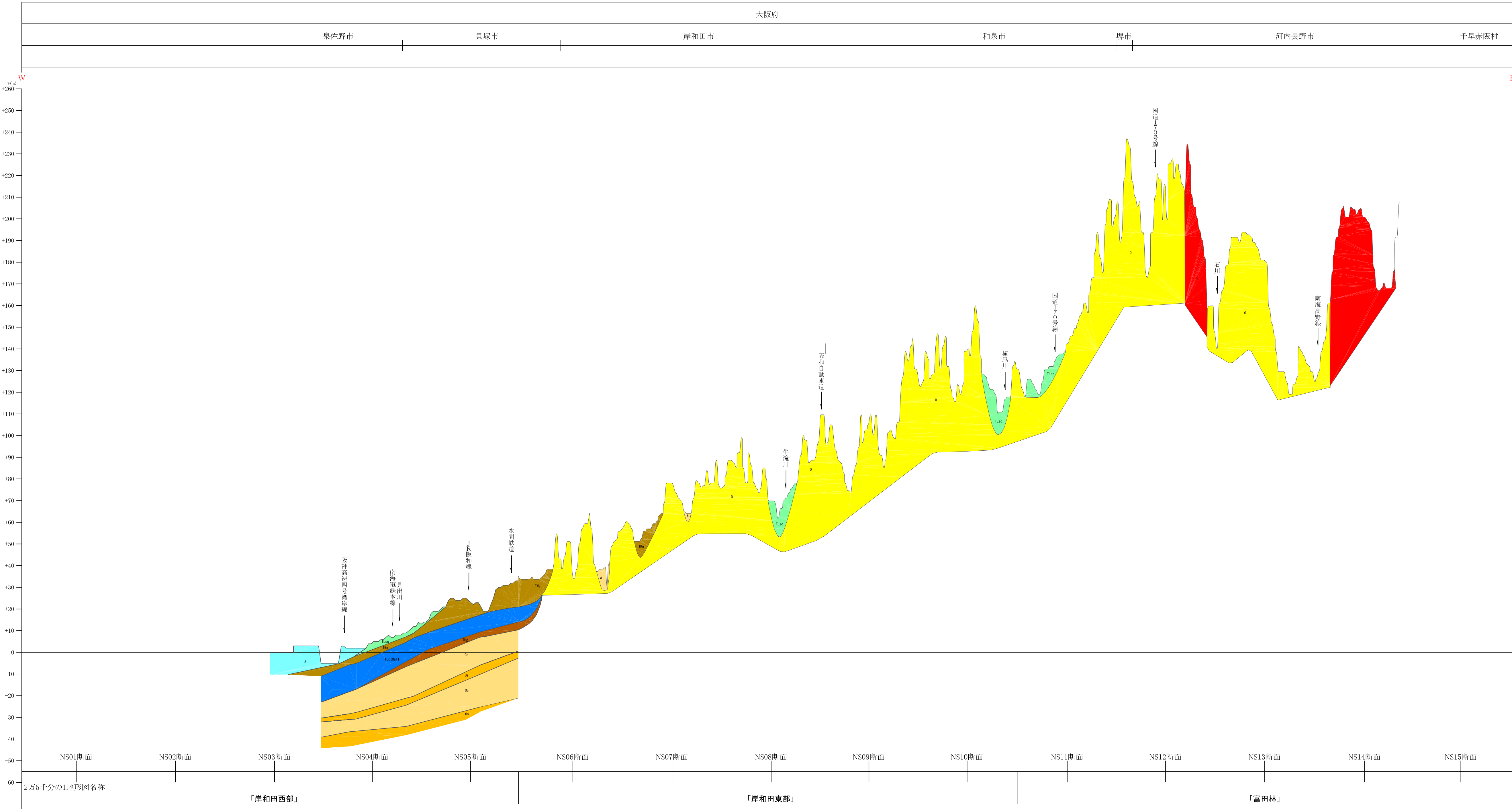
WE06断面
