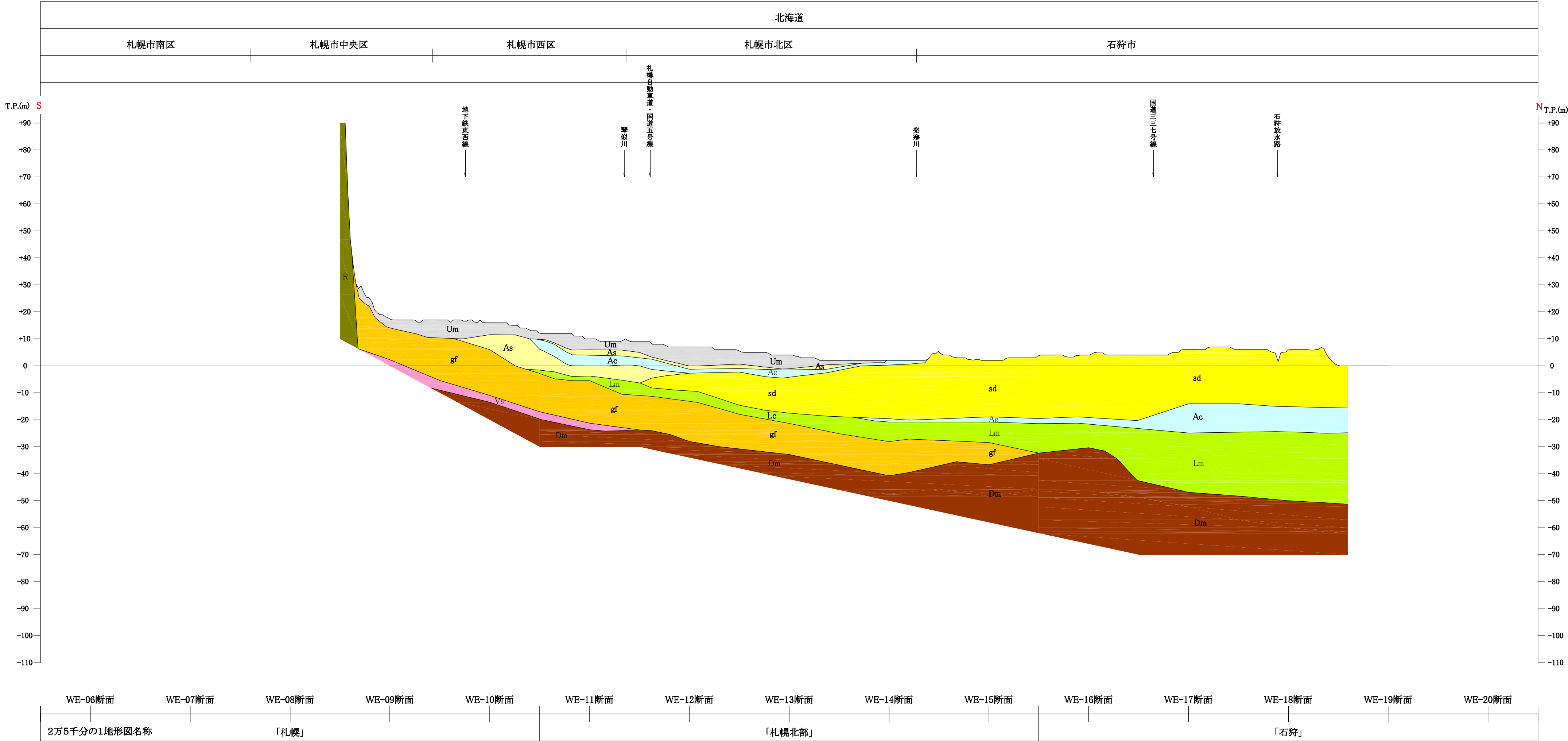
SN-07断面
