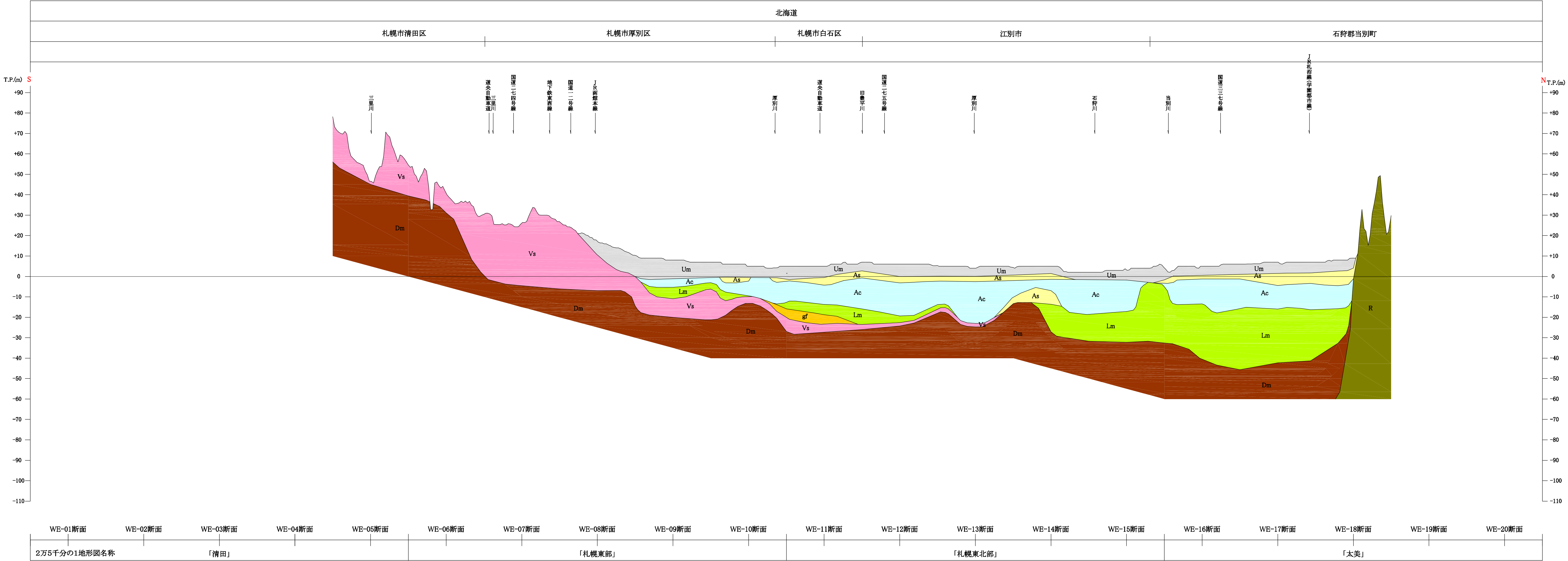
SN-13断面
