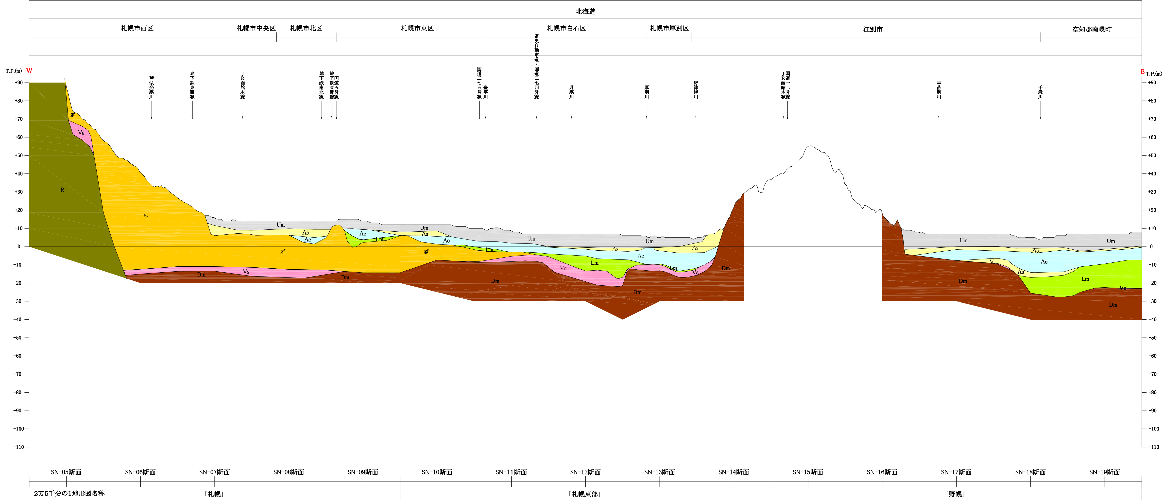
WE-10断面
