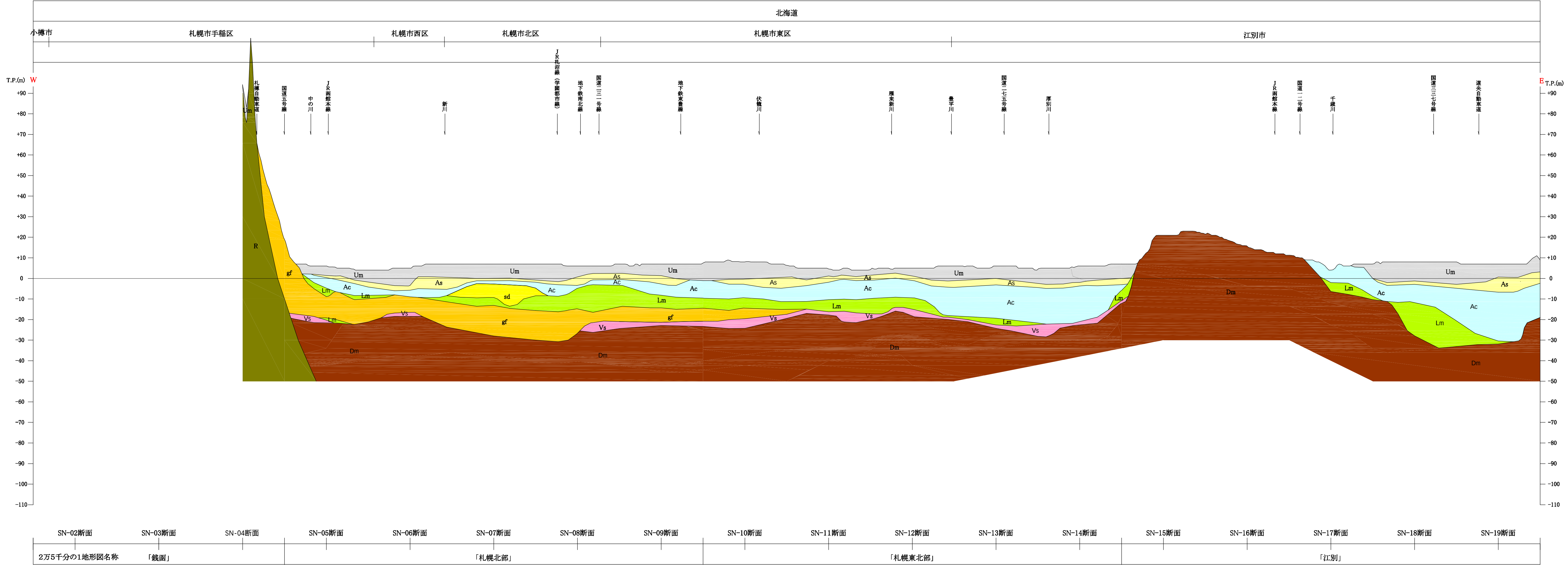
WE-12断面
