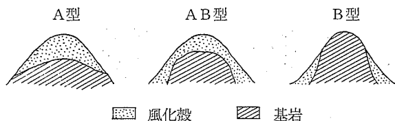
第10図 風化殻発達様式の基本型
