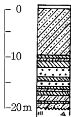
第 11 図 法勝寺川天万(手間)の柱状図 (凡例は第 12 図に同じ)
