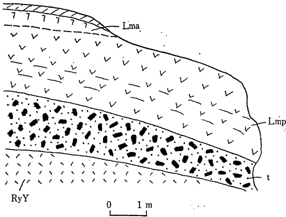
第1図 古崖錐堆積物の産状
